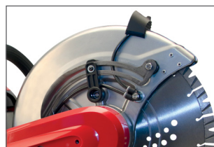
Kit d'arrosage
