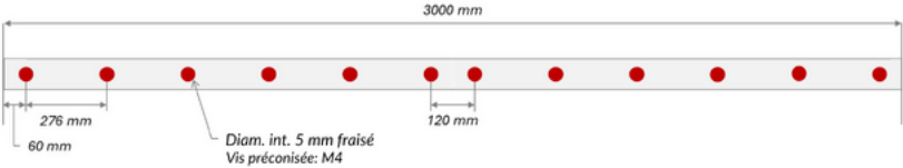
Ref 810399. Entraxe de perçage 27.6 cm, 12 trous, longueur 3 m (en option) :
